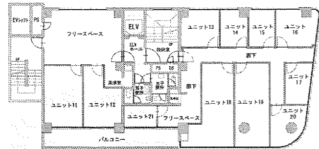
3階平面図
